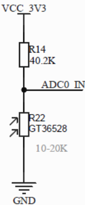
光敏电阻
